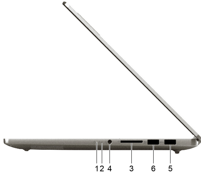
Figuur 7. Rechterkant-IdeaPad Pro 5 14IRH8, IdeaPad Pro 5 14ARP8 en IdeaPad Pro 5 14APH8
